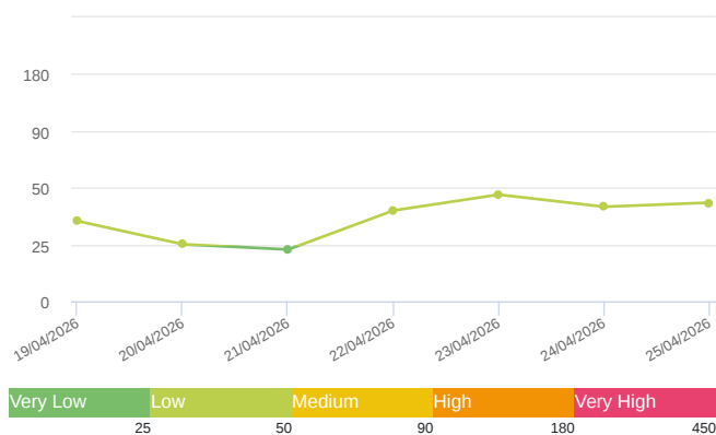
NO 2 (μg/m 3 )
