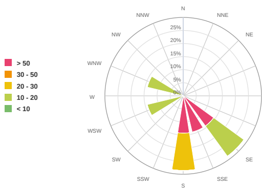
Temperature (°C)
